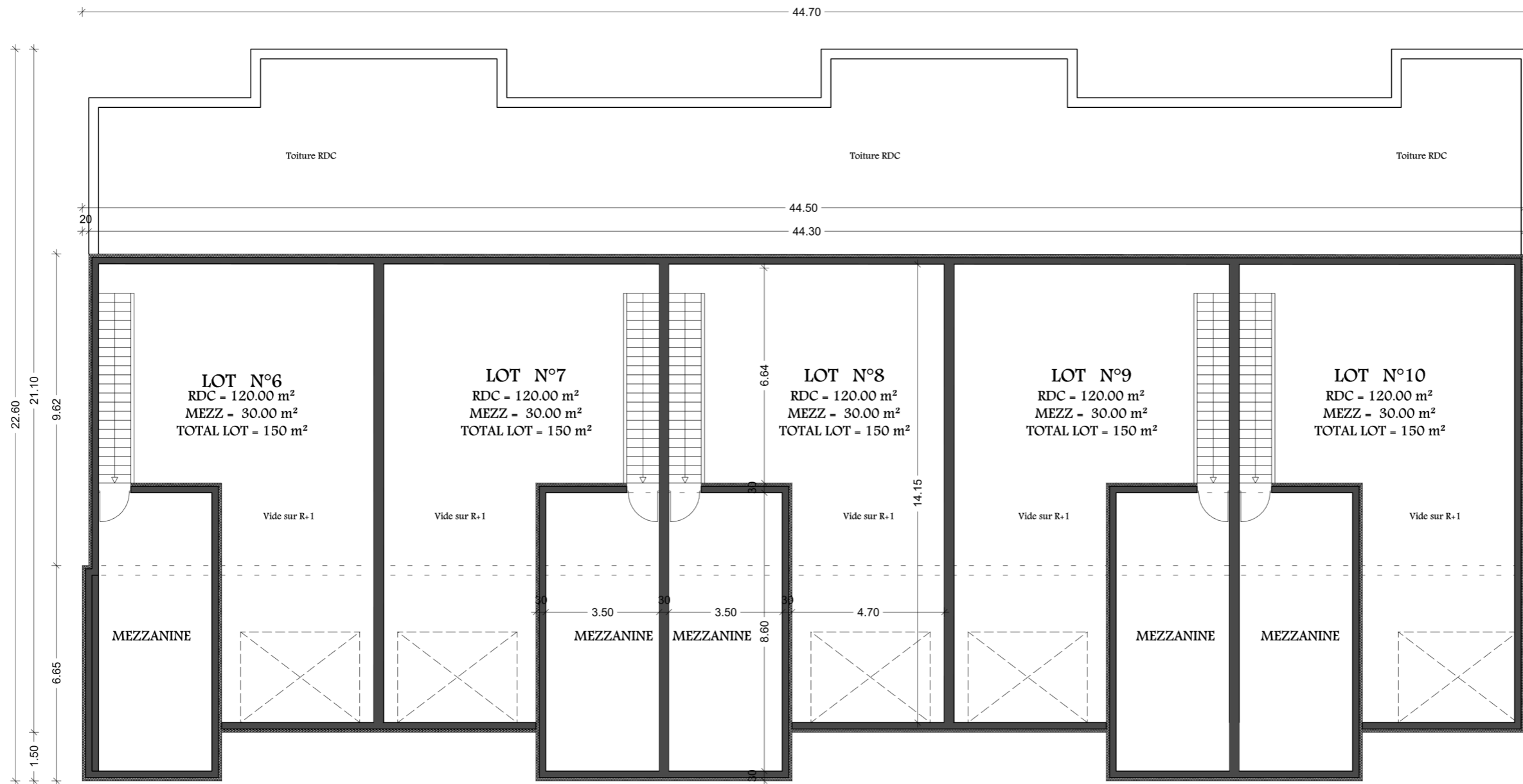
PLAN MEZZANINE DU R+1
